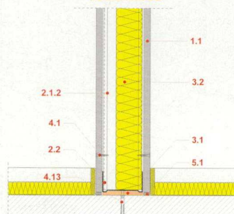
Szerelt fal csatlakozása nyers födémhez
