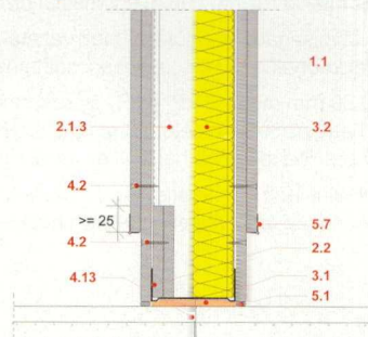
Szerelt fal redukált csatlakozása padlóhoz a tűzvéde mi és akusztikai tulajdonságok megtartásával
