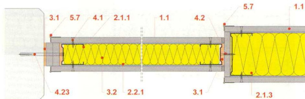
Szerelt fal csatlakozása oszlophoz, falvékonyítással, árnyékhorronnyal
