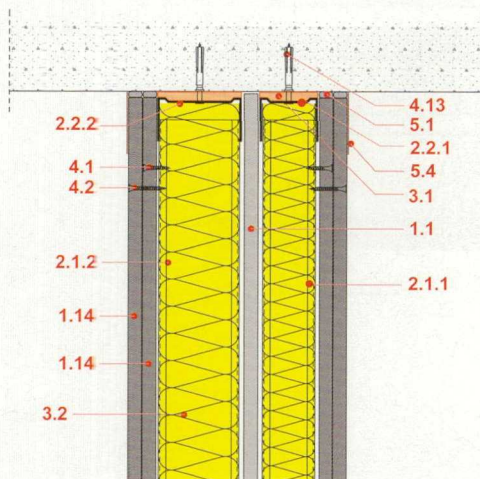
Lakésválasztó fal csatlakozása mennyezethez
