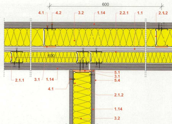
Lakésválasztó fal T csomópontja
